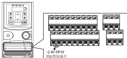
图 3-12 U 型短接位置示意图
