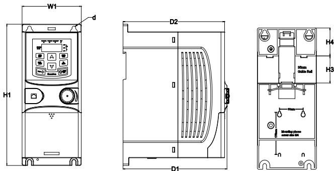
图 B-5 单相 220V/三相 380V 2.2kW(含)/ 三相 220V 0.75 kW (含)以下以下导轨安装示意图
