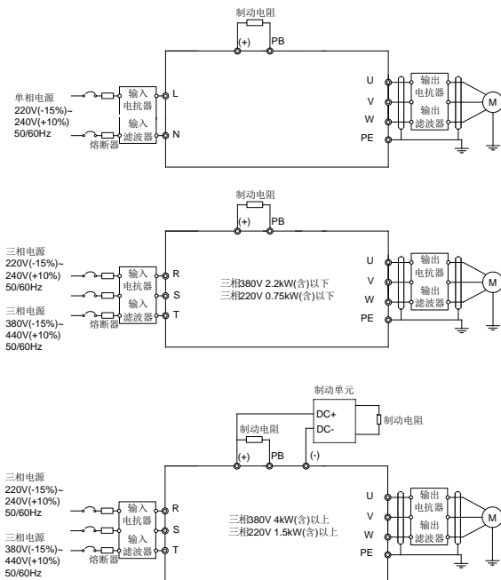
图 3-3 主回路接线图
