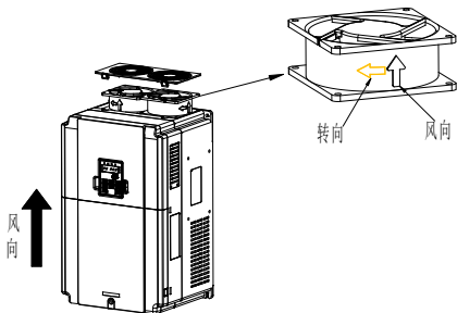
图 6-2 三相 380V 4kW (含) 以上机器风扇维护示意图
